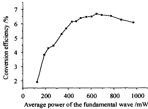
图 3 转换效率随抽运波长的变换曲线
