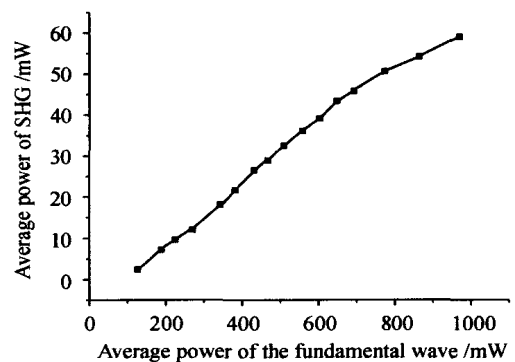
图 2 二次谐波输出功率随抽运功率的变化曲线
