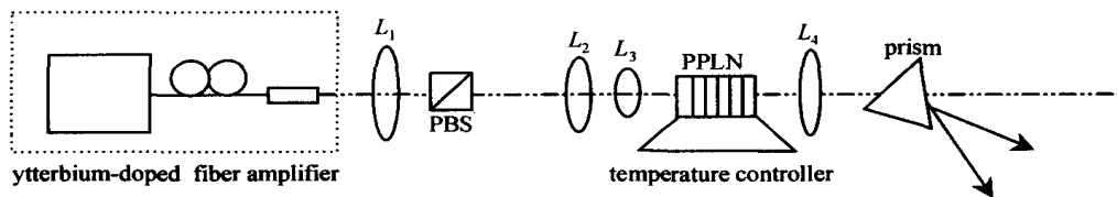
图 1 实验装置
