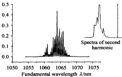
图 4 基波和谐波频谱
